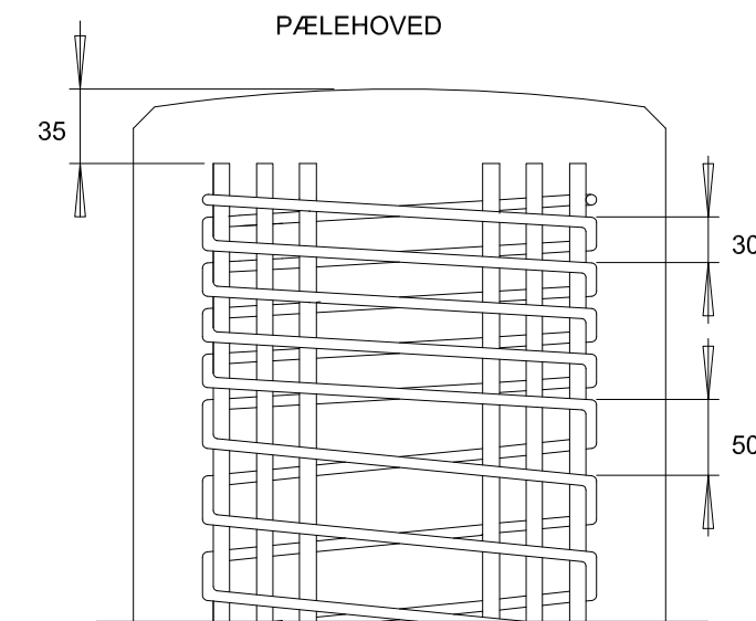
⑥ Forstærkningsbøjle ved pæleende
